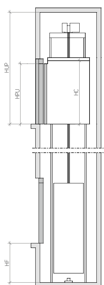
SEZIONE VERTICALE
